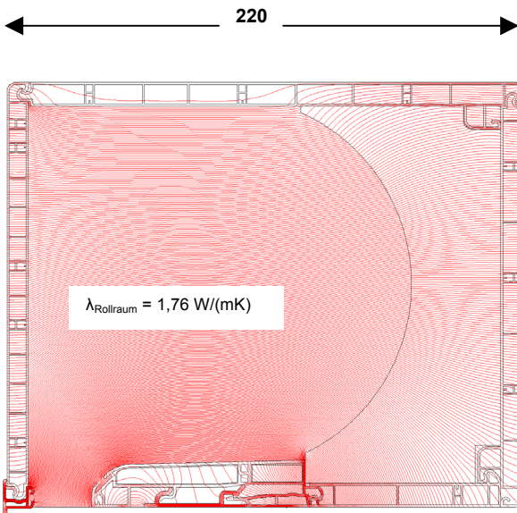
Rollladenkasten 180 x 220, Rev. unten Verlauf der Wärmestromlinien
